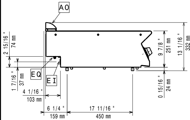
侧视
